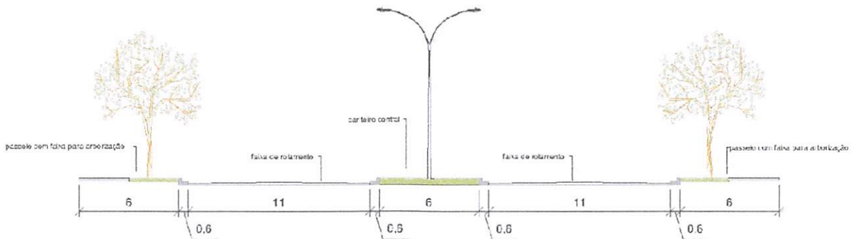
Calçada (6m) – Faixa de Rolamento (11m) – Canteiro Central (6m) – Faixa de Rolamento (11m) – Calçada (6m)
