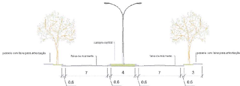
Calçada (3m) – Faixa de Rolamento (7m) – Canteiro Central (4m) – Faixa de Rolamento (7m) – Calçada (3m)
